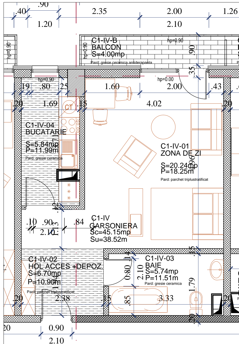
Corp C1 - etaj 2 - Apartament IV
